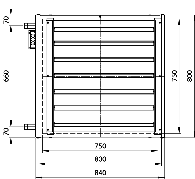
Vorderansicht
