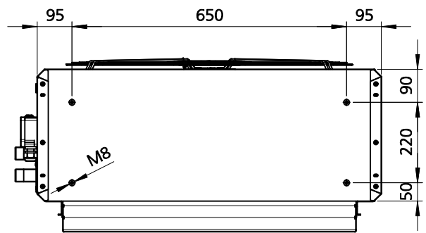
Befestigungsbohrungen
